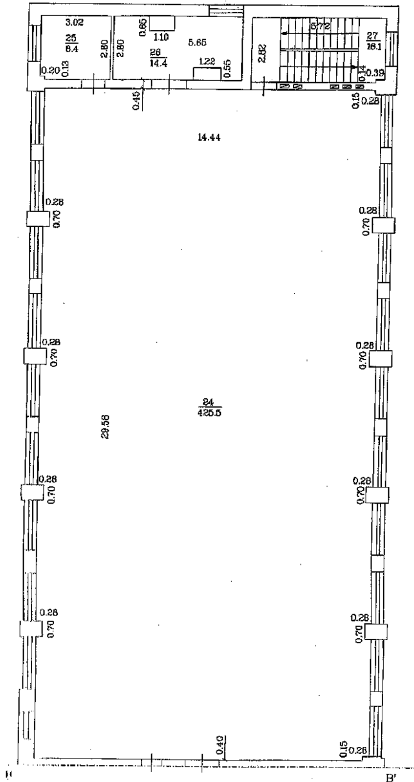
Būves daļējuma shēma
